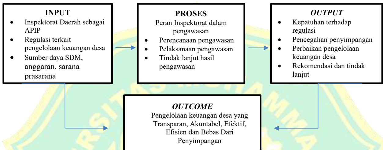
Gambar 2.3 Kerangka Konseptual
