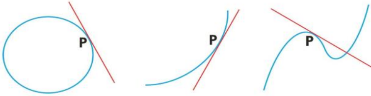
Gambar 2.1 Garis Singgung (Sumber : Djohan & Budhi, 2008)
