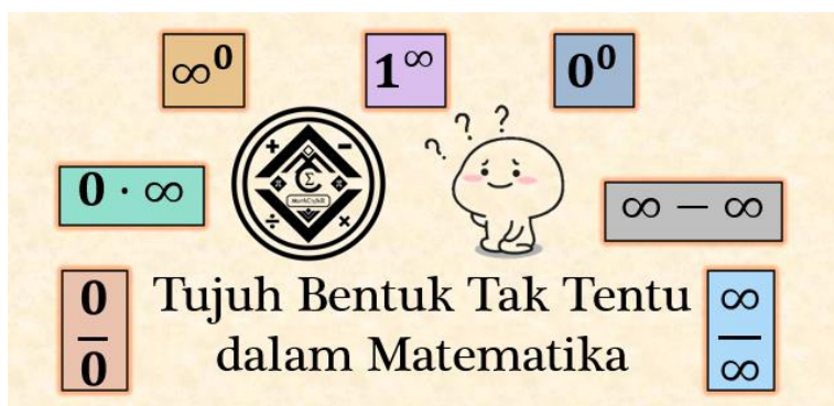
Gambar 5.2 Tujuh Bentuk Tak Tentu dalam Matematika
