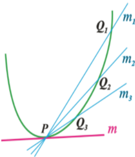
Gambar 2.2 Garis Singgung (Sumber : Djohan & Budhi, 2008)
