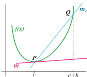
Gambar 2.3 Garis Singgung (Sumber : Djohan & Budhi, 2008)
