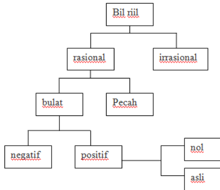
Gambar 1. Diagram Pohon Bilangan
