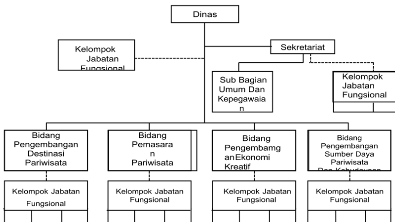
Gambar 4.1 Struktur Organisasi
